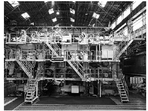
板紙向けプレスパート (MJ プレス)
