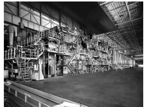
上質コート紙抄紙機 MH シリーズ
