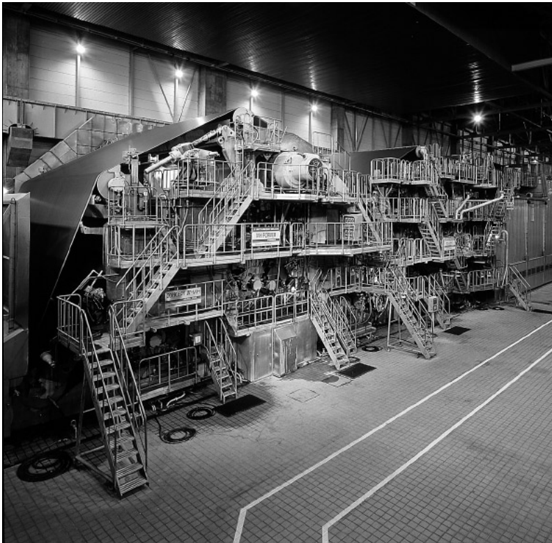
新聞用紙抄紙機 MH シリーズ
