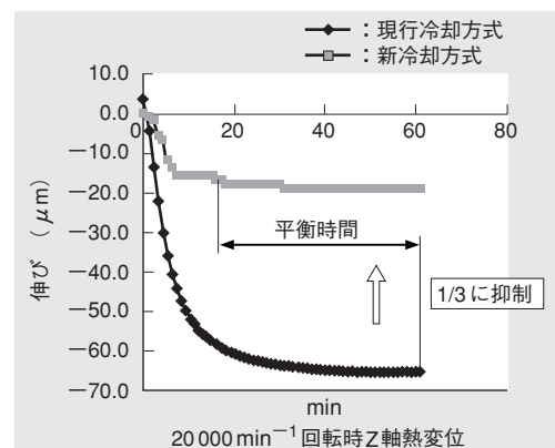
図2 主軸Z軸方向熱変位量
