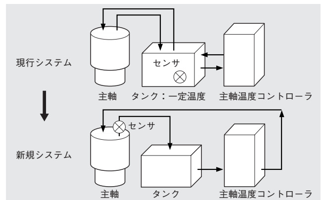
図1 主軸冷却回路図
