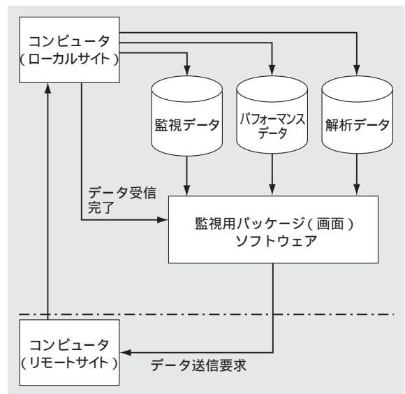
図2 ソフトウェアインターフェース
