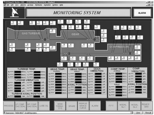
図5 監視画面の1例
