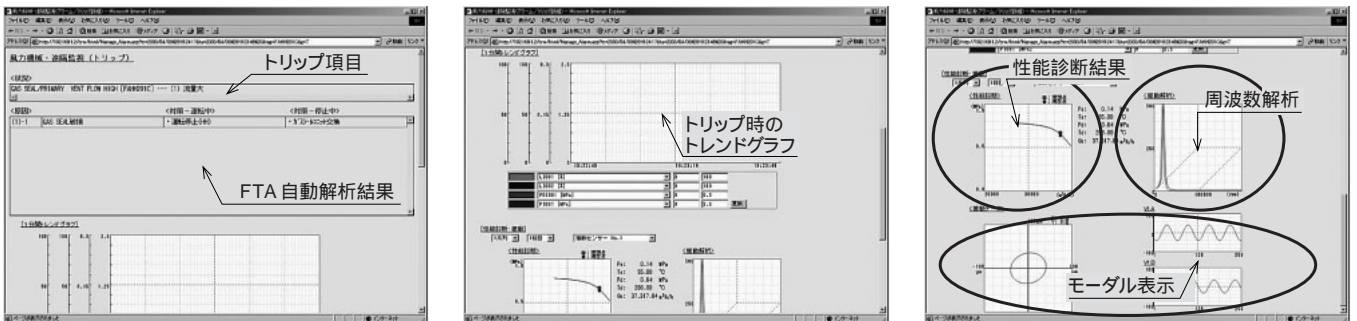
図8 振動解析，性能診断画面の1例
