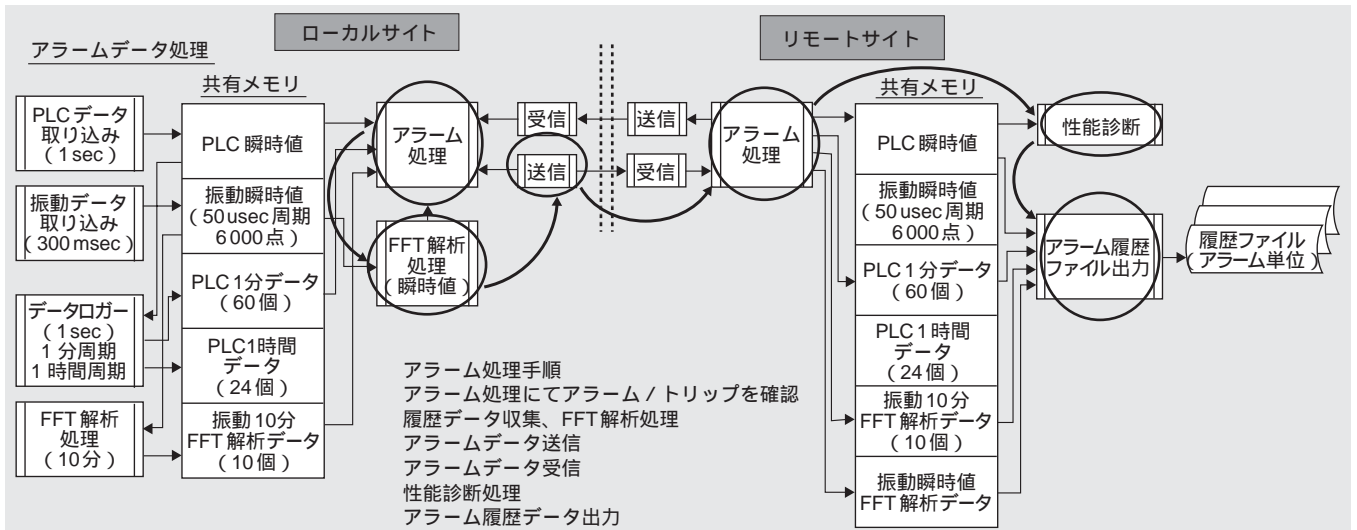
図6 異常検知時のデータフロー
