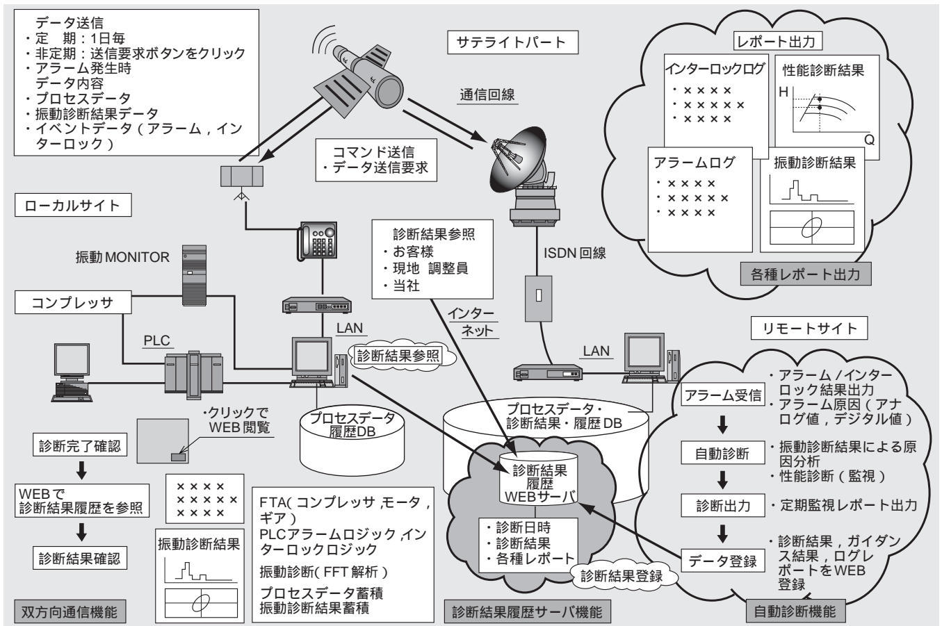
図1 遠隔監視診断システム概要
