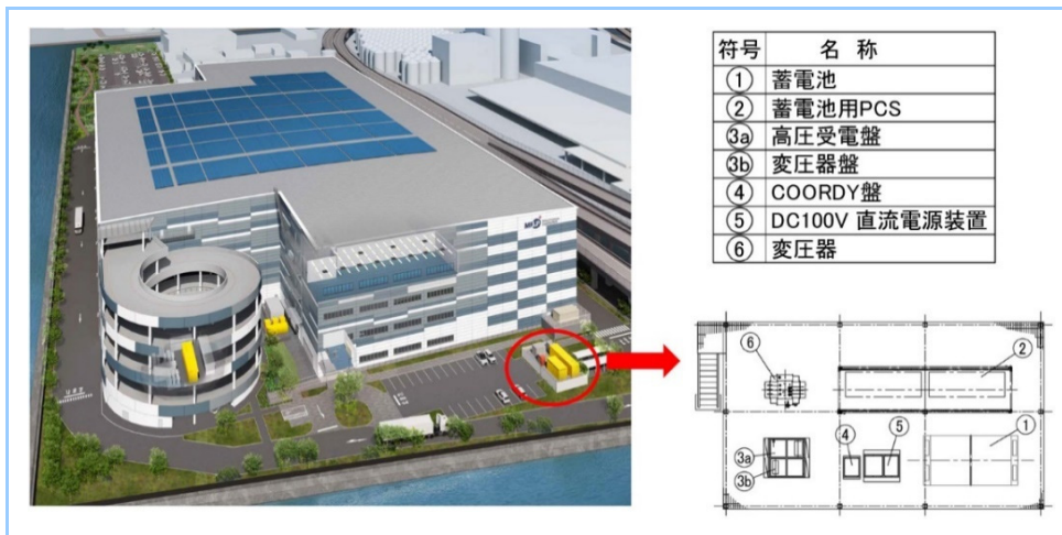
図4 三井不動産株式会社 ENEOS 不動産株式会社向 EBLOX 計画イメージ及び配置図 EBLOX(登録商標第6213361号)、COORDY(登録商標第6213362号)は、MHIETの日本における登録商標です
