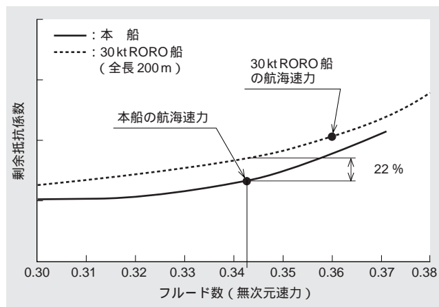
図6 剰余抵抗の比較（主船体のみ）
