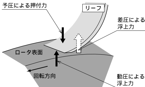
図7 リーフシール作動原理 セッティングの予圧による押し付け力、ロータ回転時動圧による浮上力、シール差圧による浮上力がバランスしてリーフが浮上する。
