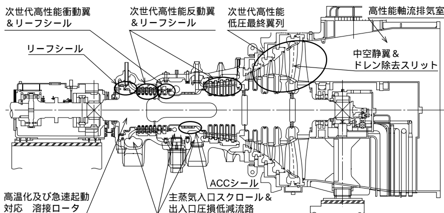
図1 高性能新形蒸気タービン（T地点向け単車室再熱タービン） 新技術の新形蒸気タービンへの適用箇所を示す。
