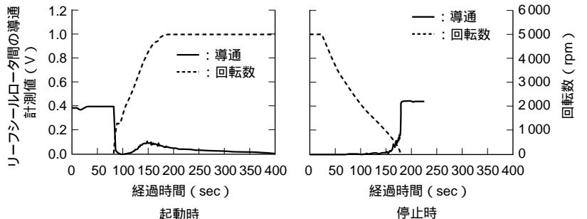
図8 リーフシール性能・浮上特性検証試験結果
