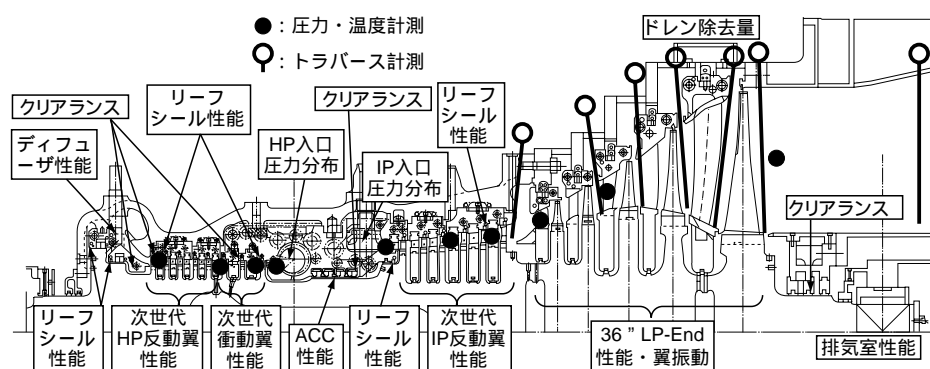
図10 T地点新形蒸気タービン特殊計測
