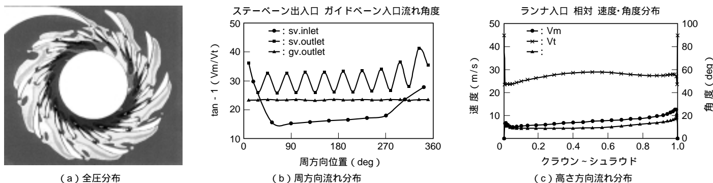
図1 ケーシング解析結果 既設機のケーシングと二重翼列の解析により、流れの非一様性を把握することができる。
