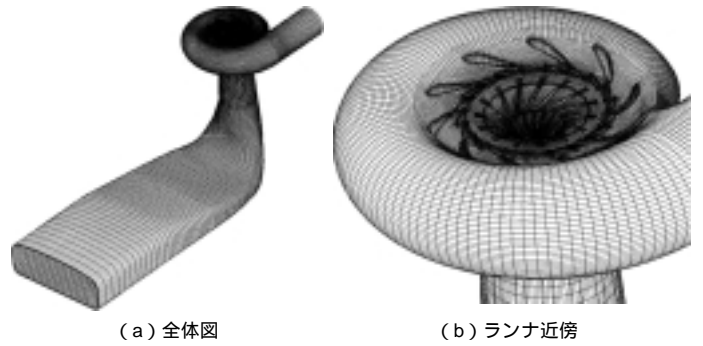
図6 一体解析用メッシュ スパイラルケーシング入口からドラフトチューブ出口までランナを含めた一体解析用のメッシュを示す。
