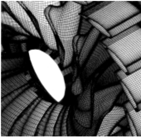
図4 翼列解析メッシュ ガイドベーンとランナの翼列解析用のメッシュを示す。予測精度向上のため壁面近傍等は細かなメッシュとしている。
