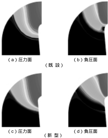
図5 静圧分布予測結果 既設ランナの負圧面シュラウド圧力が低下しているが新型ランナではこれが改善されている。
