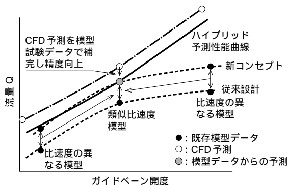
図8 ハイブリッド性能予測 新型ランナ適用後の水車性能予測はCFD解析及び類似比速度の既存モデル試験データの両面から実施した。
