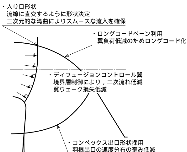
図2 設計コンセプト説明 新ランナに適用した性能向上のためのコンセプトを示す。
