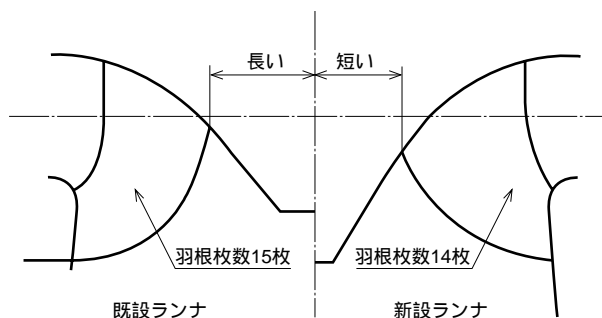
図3 子午面形状比較 既設ランナと新ランナの子午面形状の比較を示す。翼枚数を低減する一方でコード長を伸ばし負荷をコントロールし低損失化した。
