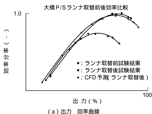
図9 現地性能試験及びハイブリッド予測結果との比較 ハイブリッド予測結果もよく一致することが分かった。
