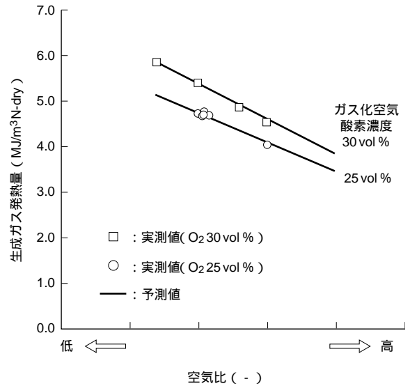
図4 24 t/d ガス化炉ガス化性能 生成ガス発熱量の実測値は予測値と良く一致している。
