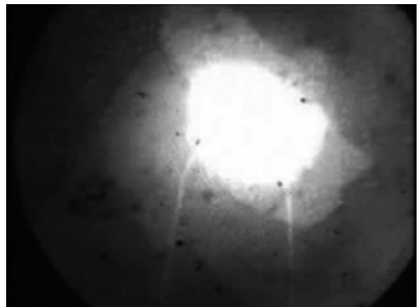
図5 24 t/d ガス化炉スラグ排出状況 スラグの排出状況は良好である。
