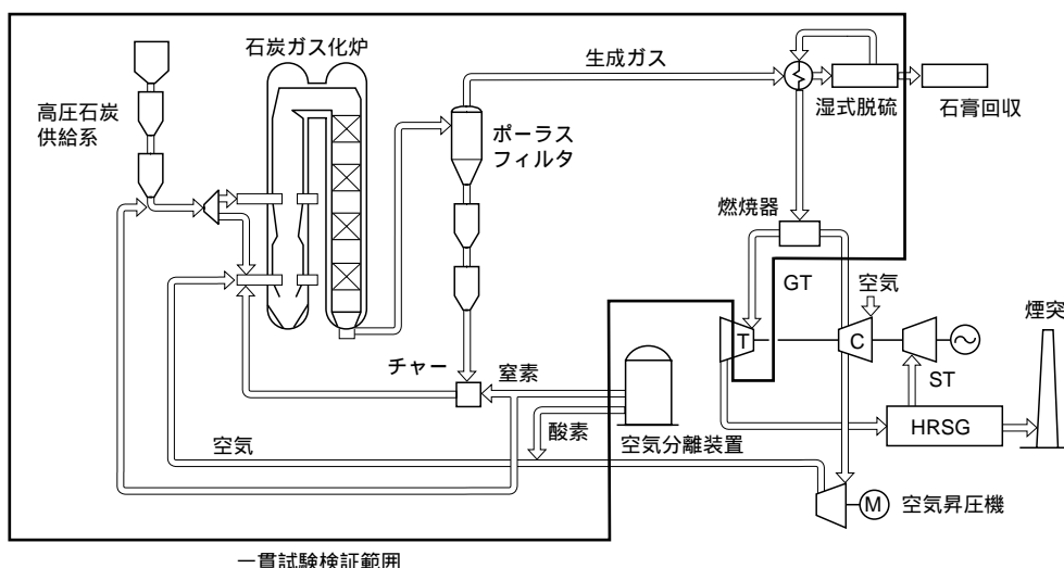
図1 IGCC実証プラントシステム 実証プラントの機器構成を示す。太線内は一貫試験設備による検証範囲を示す。
