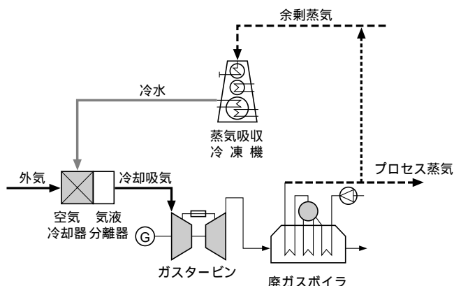
図1 吸気冷却システム概略フロー
