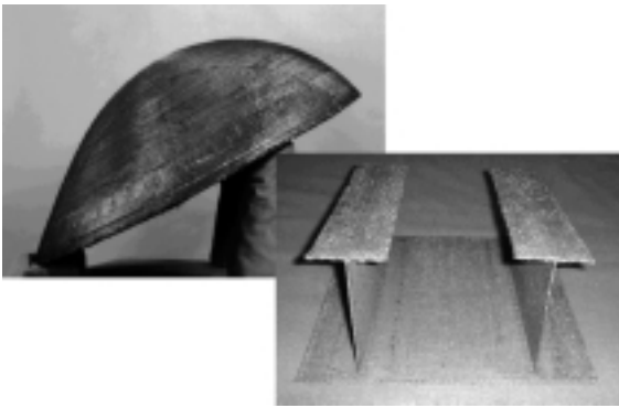
図6 HOPE-X ノーズコーン試作(製織工程時)(左図), 舵面模擬用補強平板モデル(右図) HOPE-X用C/C ノーズコーン試作品と舵面を想定して試作した補強平板モデルを示す。
