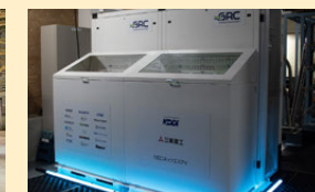
液浸冷却装置 (室内)
