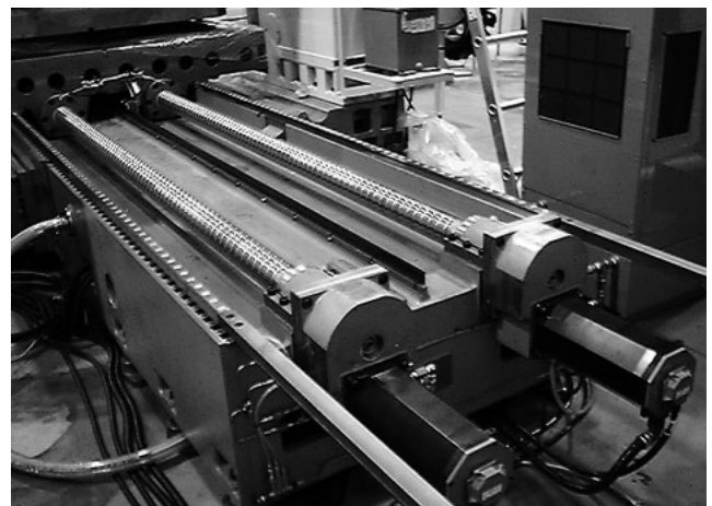
図1 X軸ツインボールネジ ベッドに2本のボールネジを取付けベッド後端のモータで駆動する様子を示す。
