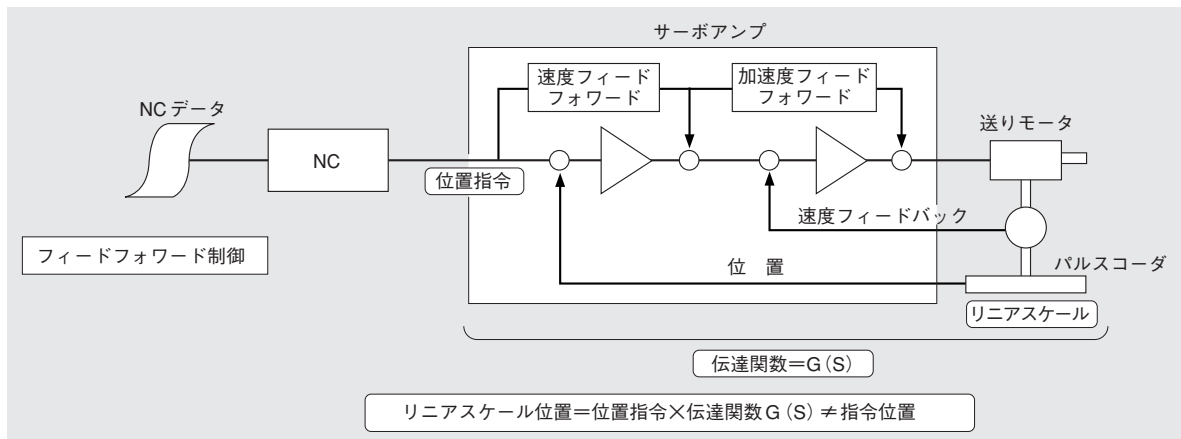
図2 フィードフォワード方式 ブロック図 フィードフォワード制御の場合。
